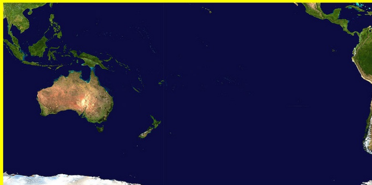
http://commons.wikimedia.org/wiki/File:Oceania_satellite.jpg
