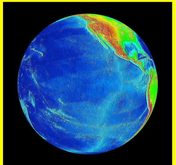
http://commons.wikimedia.org/wiki/File:Pacific_Ocean_surface_2.jpg
