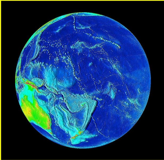
http://commons.wikimedia.org/wiki/File:Pacific_Ocean_surface_1.jpg
