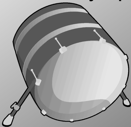
tympány
