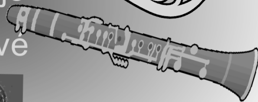
klarinet
