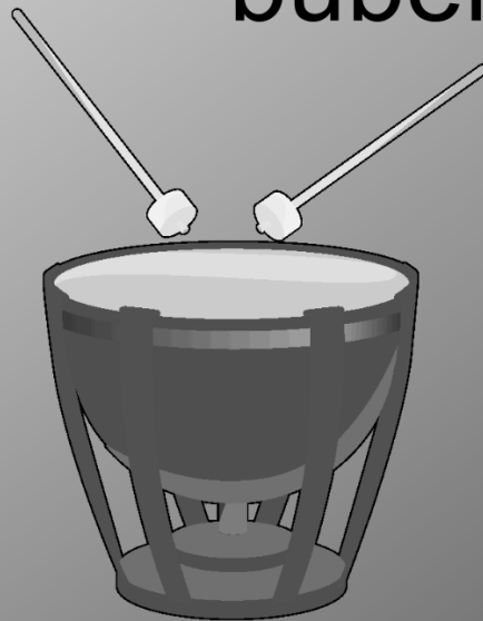
tympány
