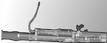
fagot
